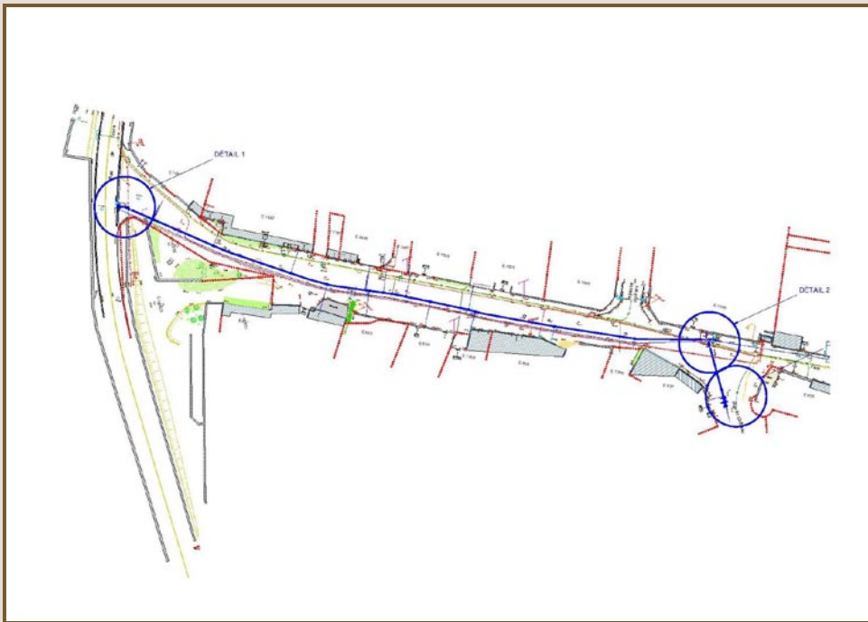
Plans de remplacement de la canalisation AEP Rue du Parc et Rue des Cerisiers
